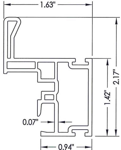
8 HANDLE STILE
